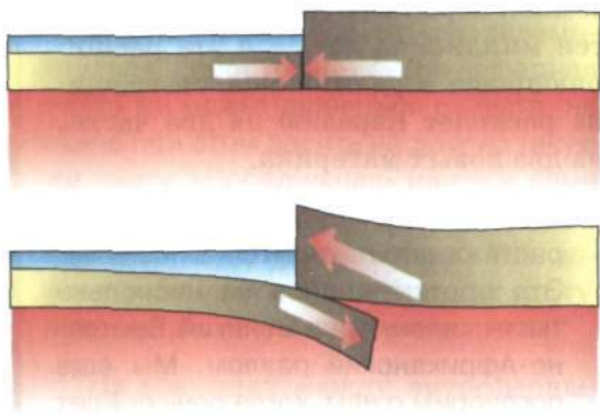
Рис. 24. Столкновение участков материковой и океанической земной коры
