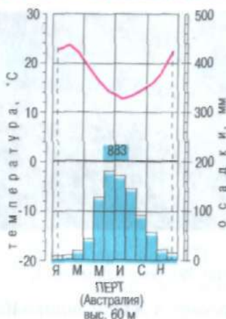
Рис. 176. Субтропический климат (климатограмма)
